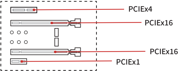
图2-4 PCI扩展插槽
